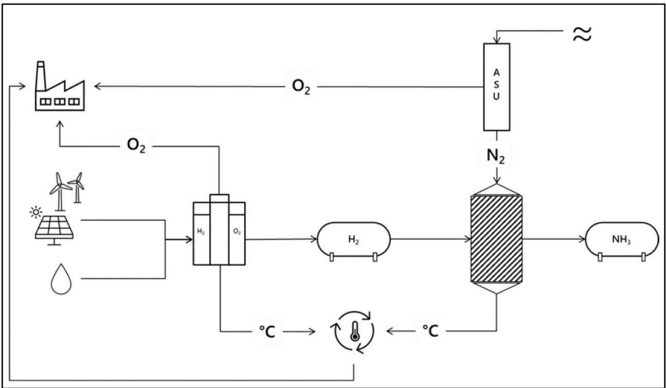
Kuva 4. Tuotantolaitoksen yksinkertaistettu prosessikaavio, jossa esitetyt kemikaalit: Vety ( H_2 ), Ammoniakki ( NH_3 ), Typpi ( N_2 ), Happi ( O_2 ) ja Argon (Ar).
